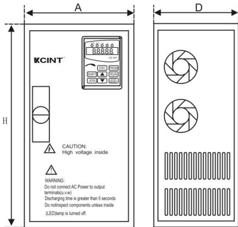
1.2.3. 外形尺寸图三:金属壳机箱（立柜式）
